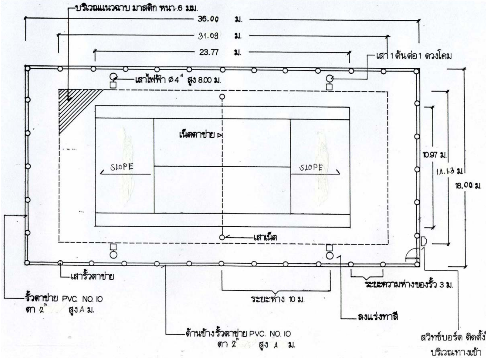
แปลนสนามเทนนิส 1 คอร์ท ขนาดมาตรฐาน SCALE 1 : 200
